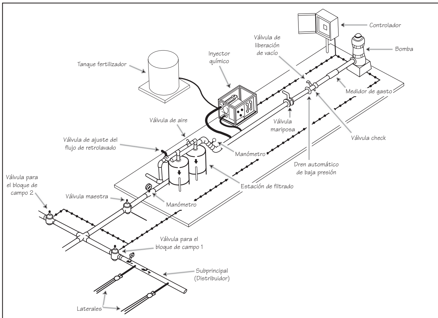
Figura 11. Trazo típico de una estación de bombeo en el que se muestra el equipo de filtración.
